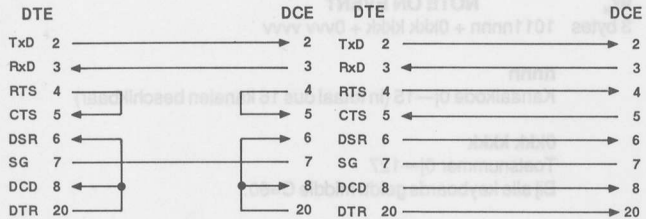
Tweedraads DTE - DCE-verbinding
