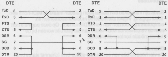
Tweedraads DTE - DTE-verbinding
